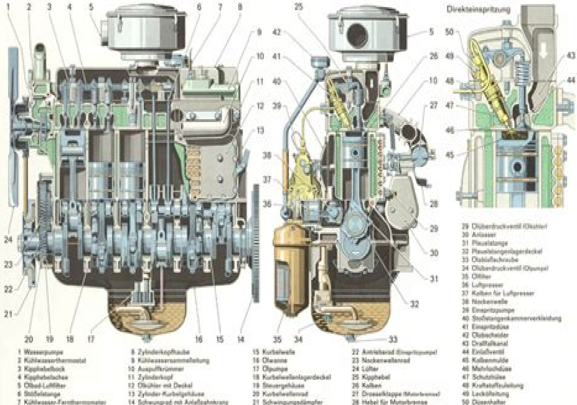
Motor-Längs- und Querschnitt OM 352
