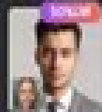
AI Avatar
